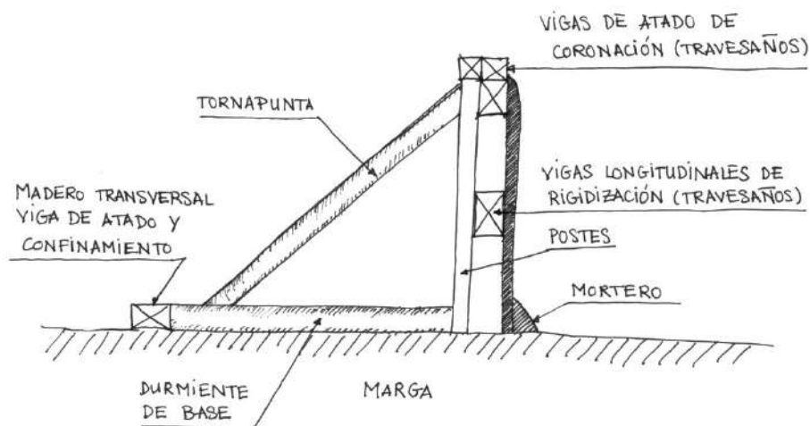
Esquema transversal del sistema constructivo del Azud de Santa Engracia.
