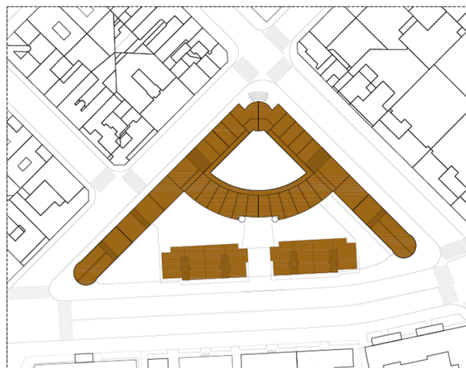
PLANTA CUARTA
